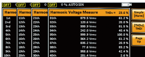
电压谐波
