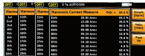
电流谐波
