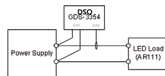
使用 GDS-3354 DSO 分别在 C.V 优先和 C.C 优先模式下测试 LED
